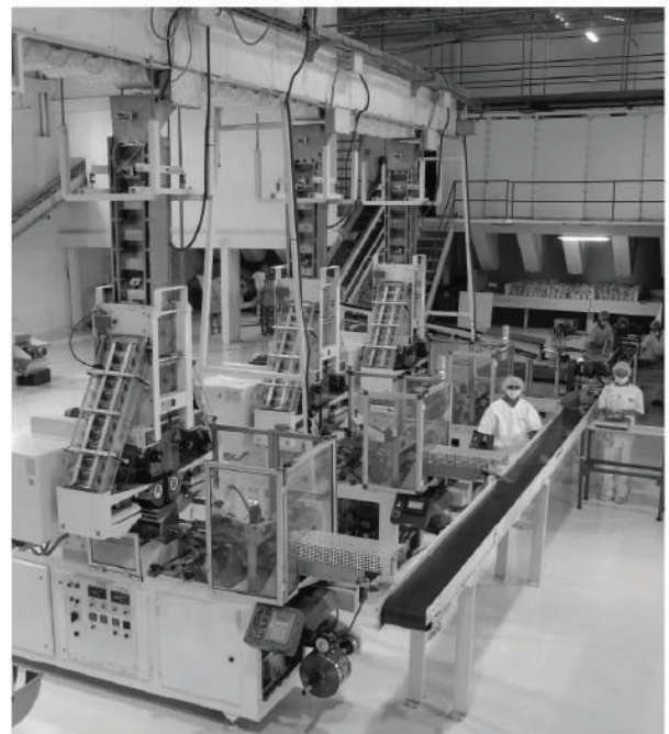
Línea de empaque de pasta larga
