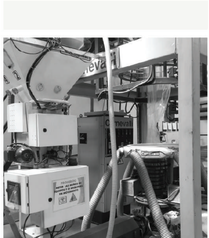
Extrusora de empaque de polietileno
