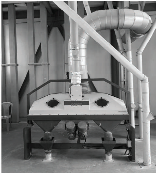
Vibroseparadora de trigo
