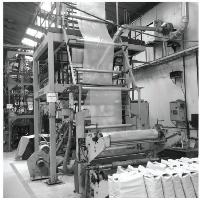
Línea de producción de lámina de polietileno
